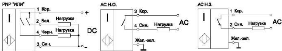
Рис. 3. Схемы подключения датчиков
