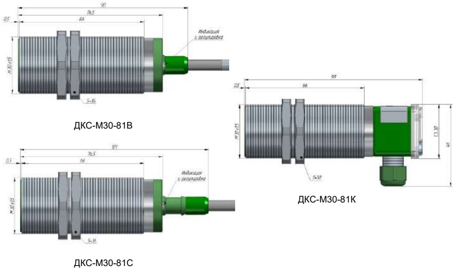
Рисунок 1 - Внешний вид и габариты ДКС
